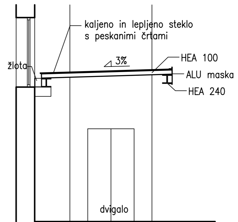
PREREZ B-B
