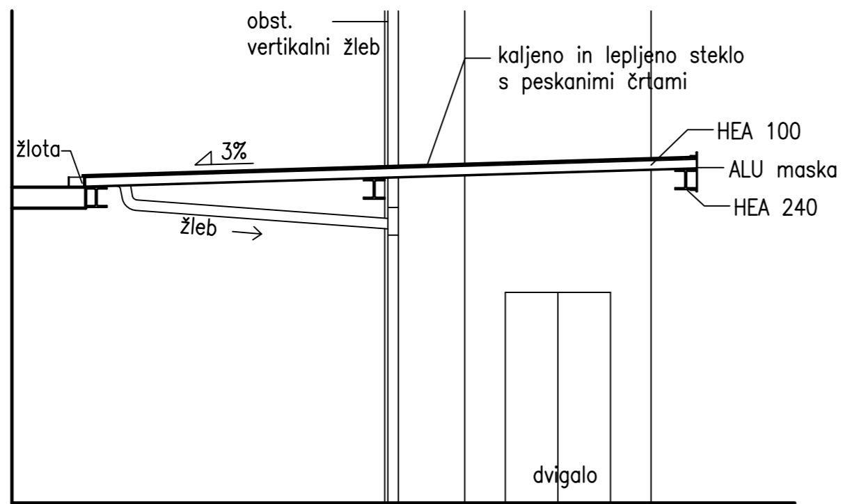
PREREZ A-A
