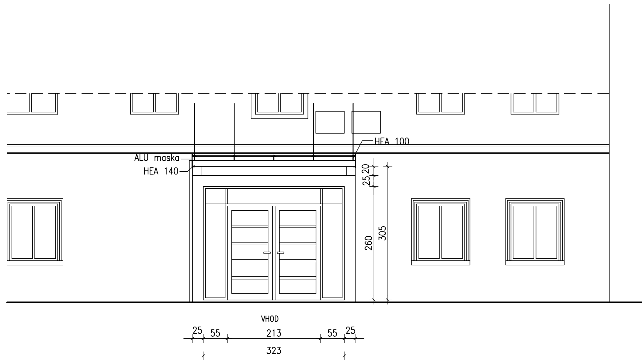
VHODNA FASADA
